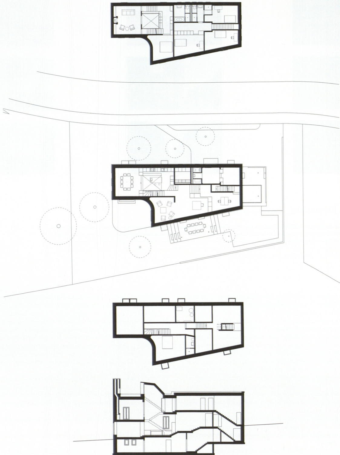
PLANTAS PRIMERA, BAJA Y SÓTANO, Y SECCIÓN LONGITUDINAL. FIRST FLOOR, GROUND FLOOR AND BASEMENT, AND LONGITUDINAL SECTION.
